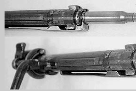
Primer plano del cerrojo del K98.
