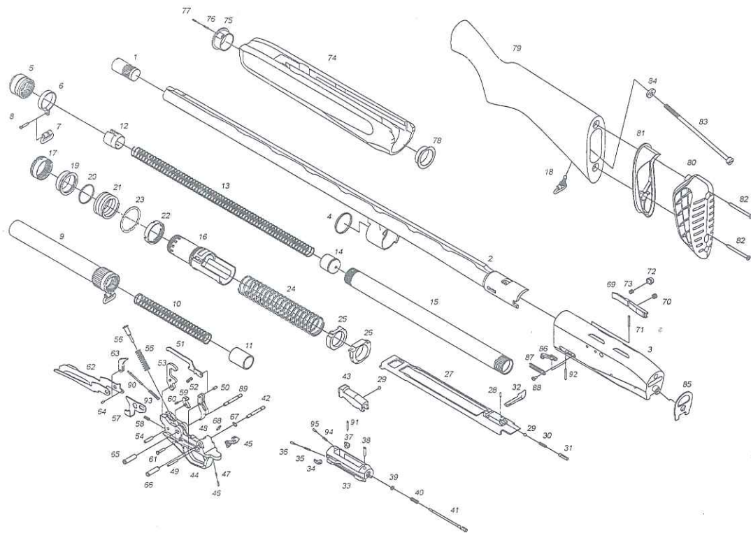
Рисунок А.2 - Сборочные единицы и детали ружья Fig. A.2 - MP-155 Exploded View
